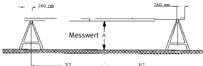
Bild 1: Unbelastete Leiter
